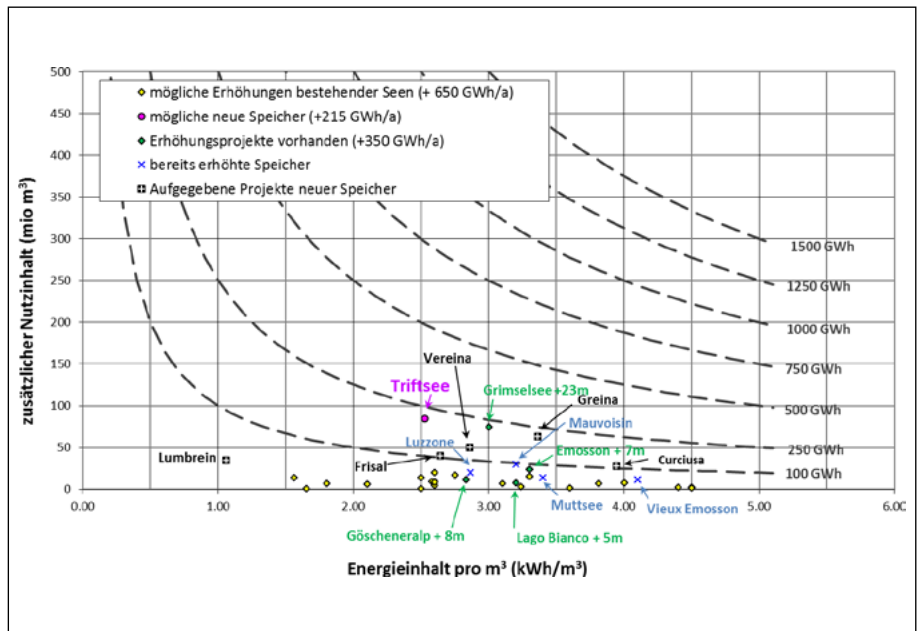
Abbildung 1: Darstellung der wichtigsten Speicherkraftprojekte (Speicherenergie in GWh) in Abhängigkeit von Energiegleichwert und Speichervolumen.
