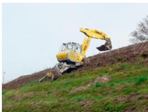
Eindrücke aus der Bauphase: Albert Steiner beim Terrassieren der Parzelle D mit einem Schreitbagger (links und mitte) und Einlegen der Bewässerungsrohre (rechts)
